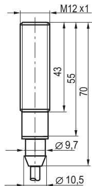
Габаритный чертеж
